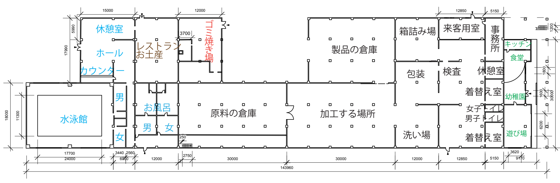
1階の平面図（水泳館+お風呂場+工場） S=1/600
