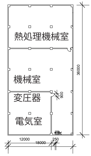
地下の機械室の平面図 S=1/600
